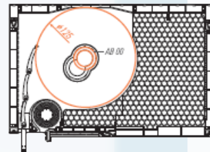
Avvolgibile monoblocco con termoisolante „TERMO” e zanzariera integrata
