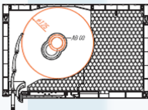
Avvolgibile monoblocco con termoisolante „TERMO”
